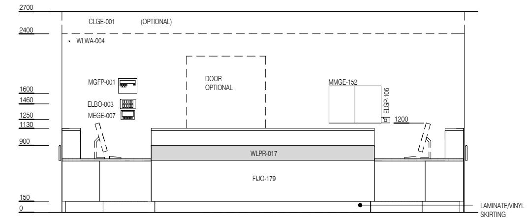
ELEVATION 2
