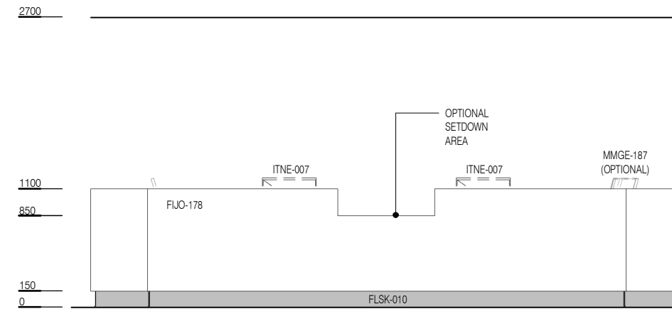
ELEVATION 5
