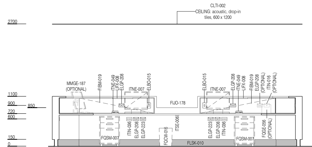
ELEVATION 4
