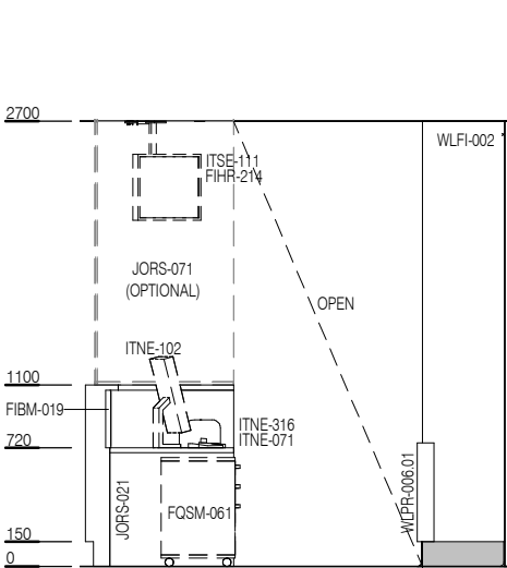
ELEVATION 1
