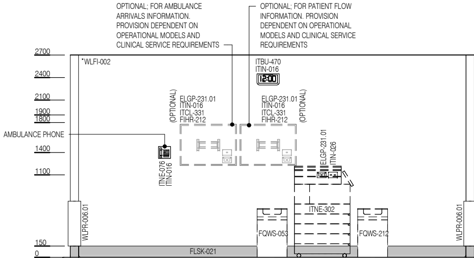
ELEVATION 2
