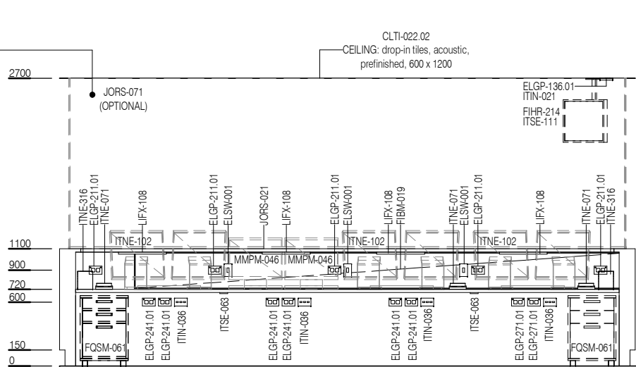
ELEVATION 4
