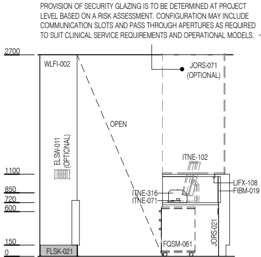
ELEVATION 3
