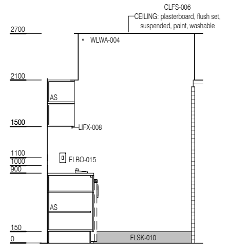
ELEVATION 2
