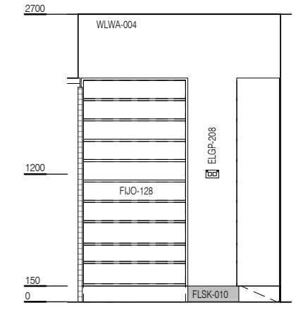
ELEVATION 4
