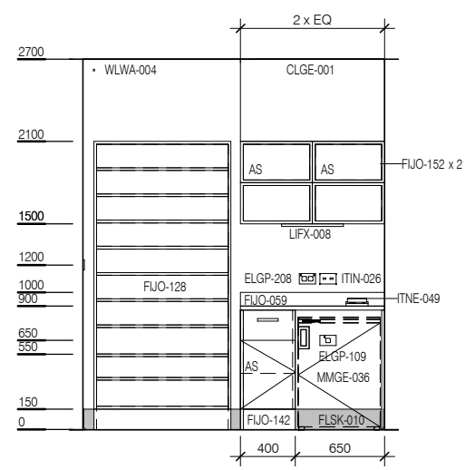
ELEVATION 1
