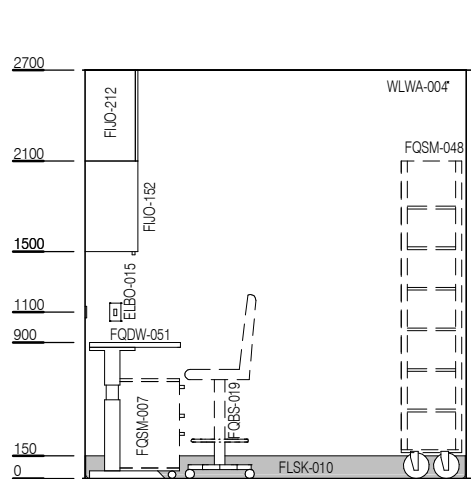
ELEVATION 1
