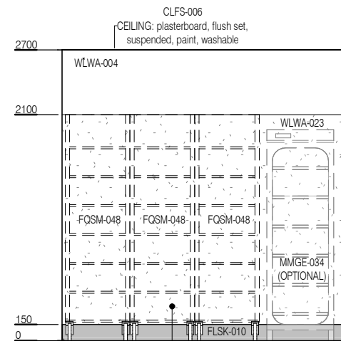
ELEVATION 2
