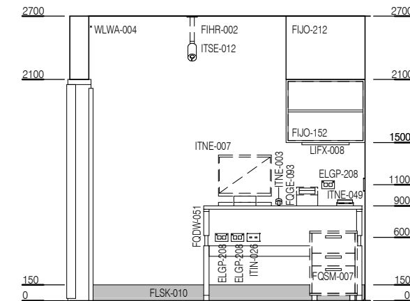
ELEVATION 4
