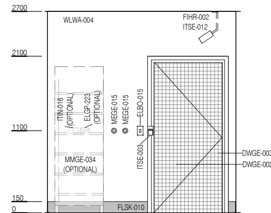
ELEVATION 3
