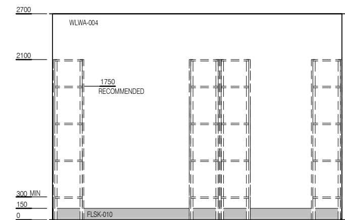
ELEVATION 4
