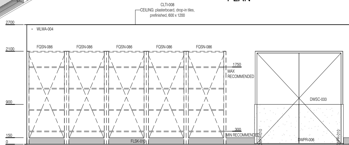
ELEVATION 1
