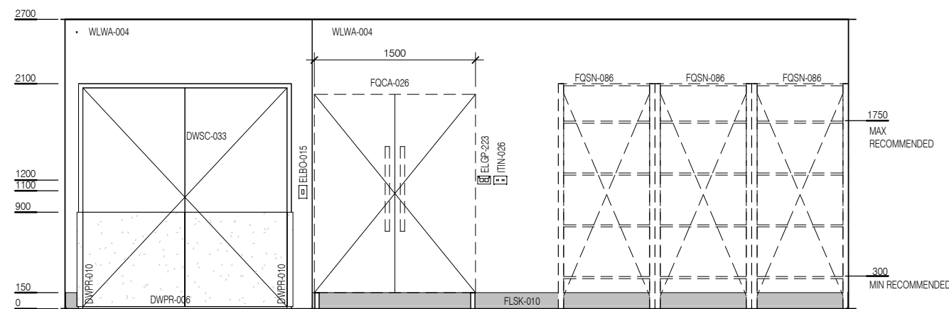
ELEVATION 3
