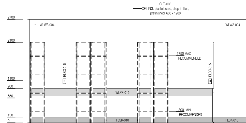
ELEVATION 2
