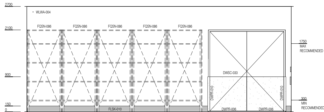
ELEVATION 1
