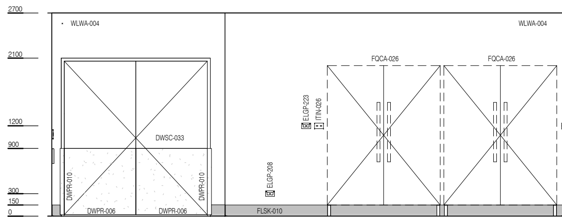
ELEVATION 3
