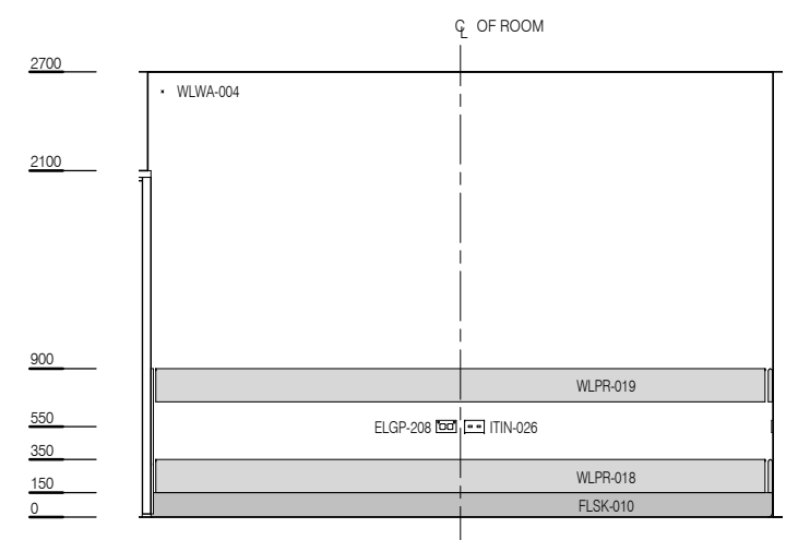
ELEVATION 4
