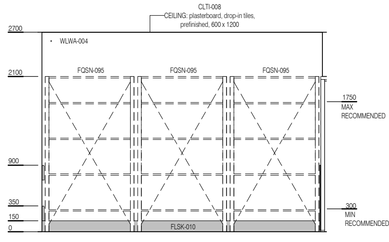
ELEVATION 2
