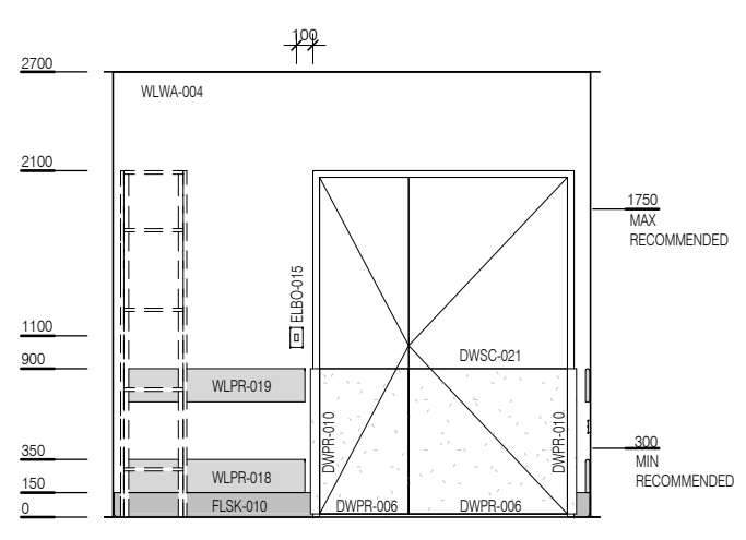
ELEVATION 3
