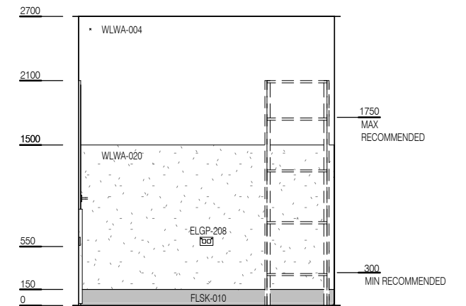
ELEVATION 4
