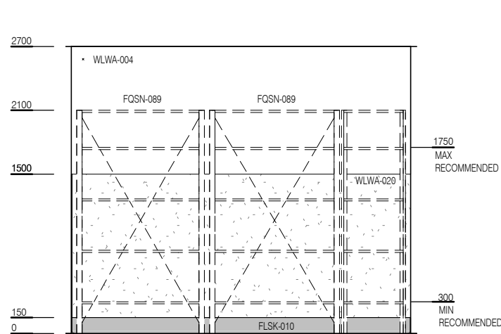
ELEVATION 1
