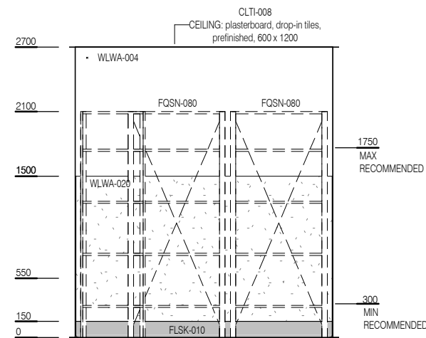
ELEVATION 2
