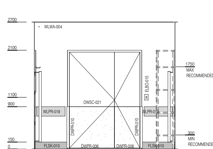
ELEVATION 3
