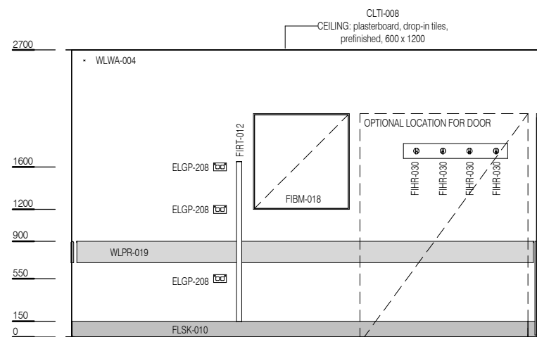
ELEVATION 2
