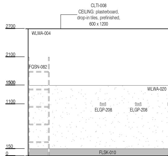
ELEVATION 1
