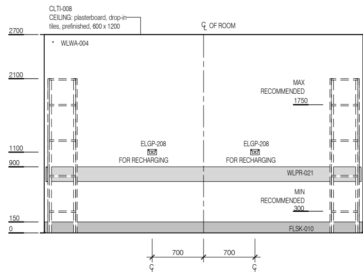
ELEVATION 1
