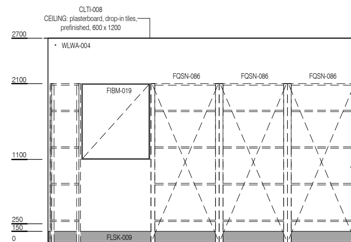
ELEVATION 3
