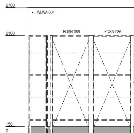
ELEVATION 2
