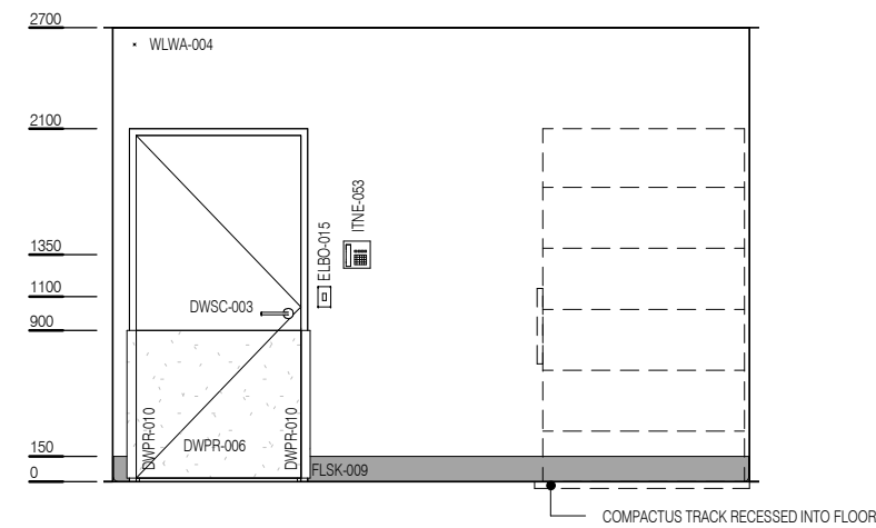
ELEVATION 3
