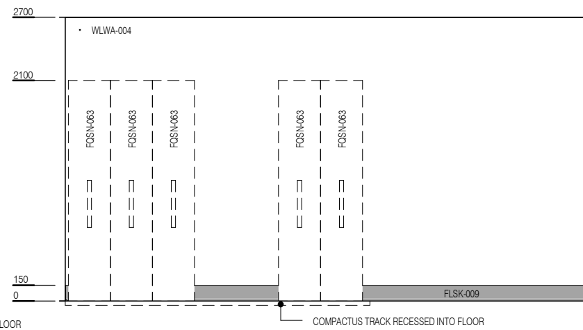
ELEVATION 2
