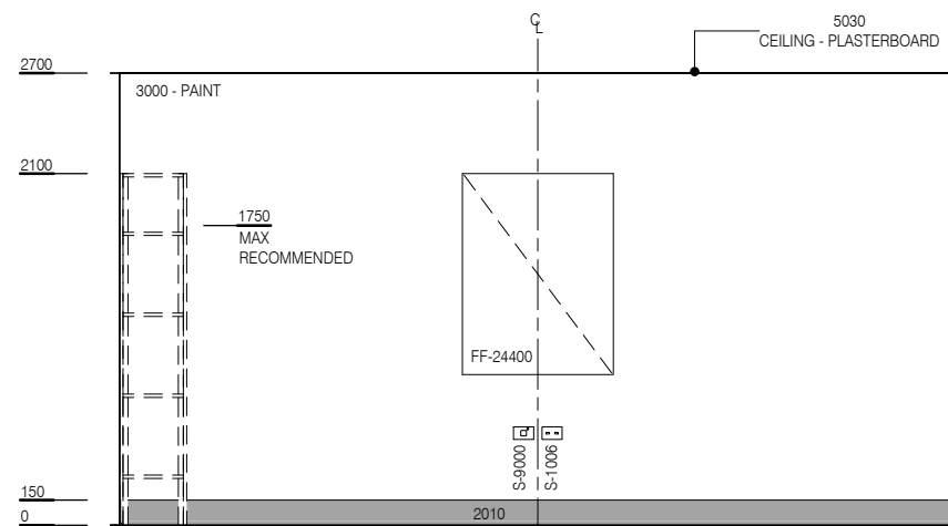
ELEVATION 2
