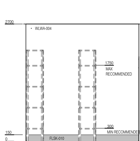
ELEVATION 1
