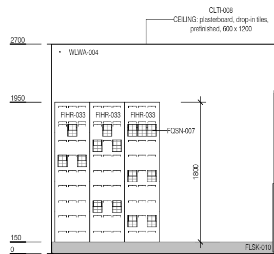
ELEVATION 2
