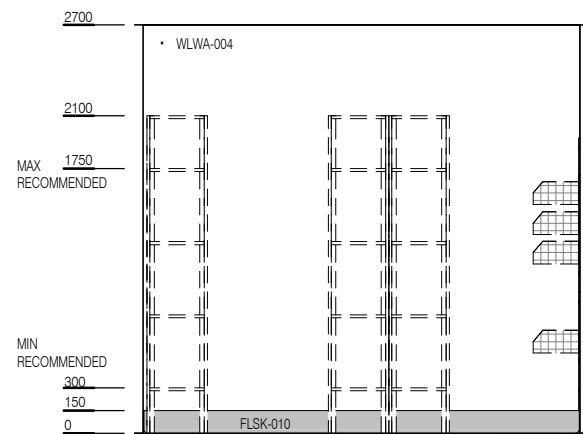
ELEVATION 1
