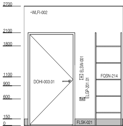
ELEVATION 3
