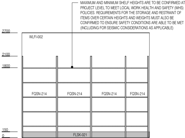
ELEVATION 4
