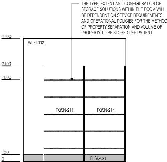
ELEVATION 1
