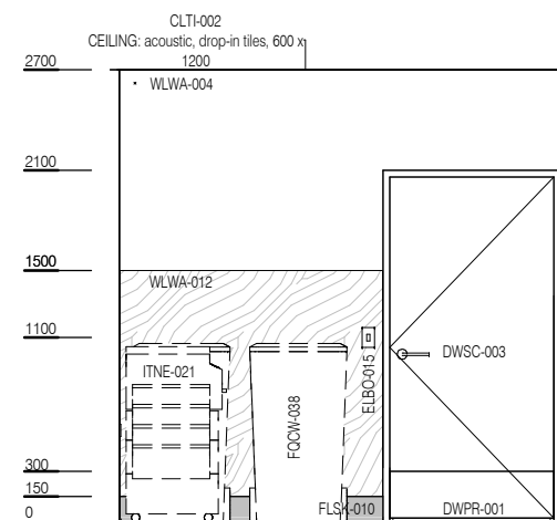
ELEVATION 3
