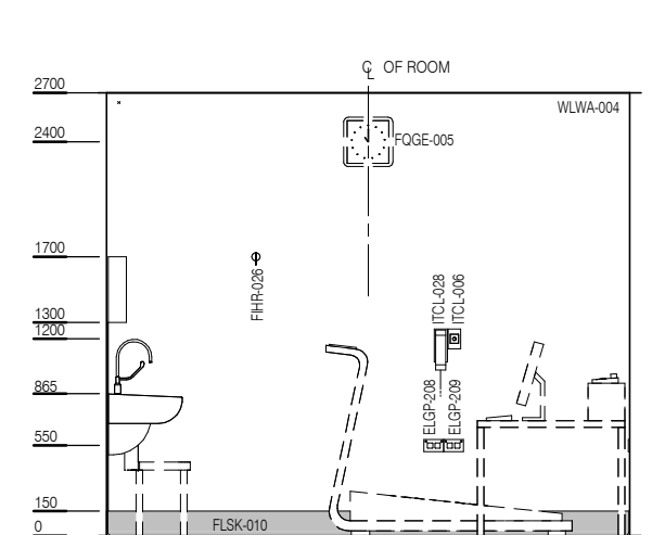
ELEVATION 4
