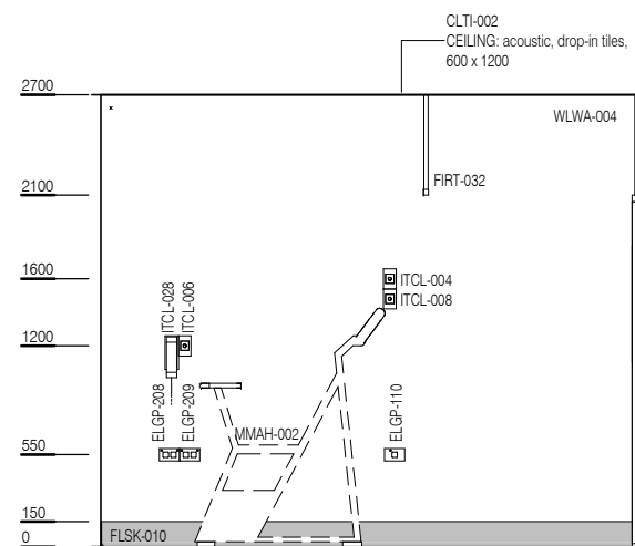
ELEVATION 2
