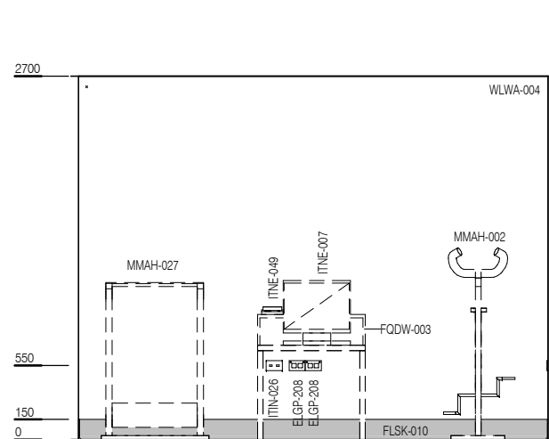
ELEVATION 1
