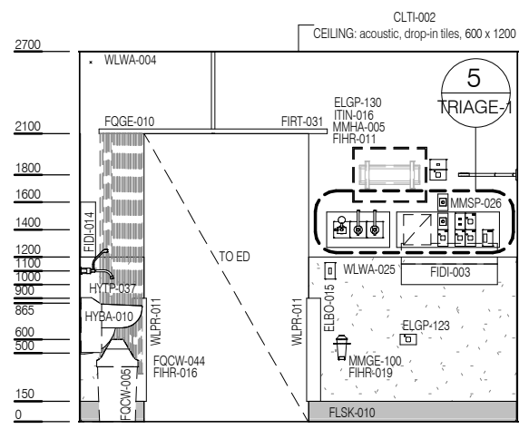
ELEVATION 1
