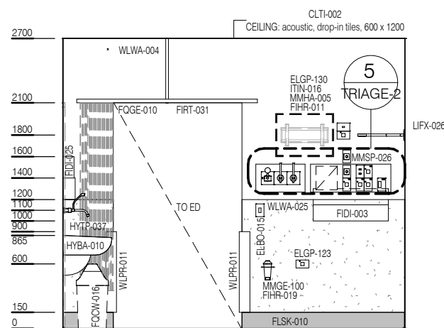
ELEVATION 1
