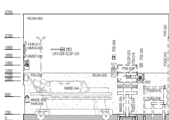
ELEVATION 2
