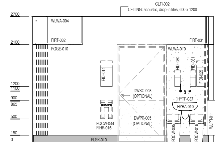
ELEVATION 4
