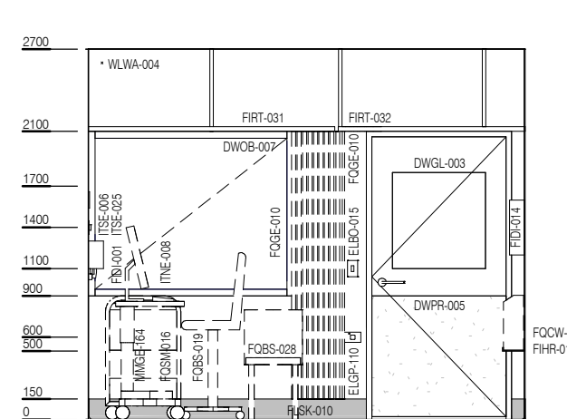
ELEVATION 3
