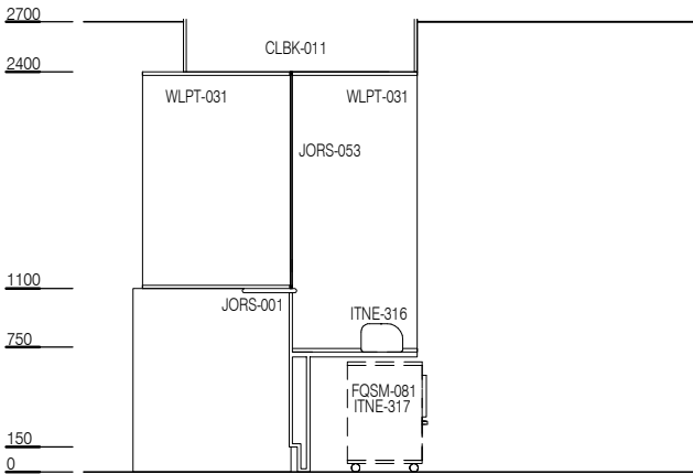
ELEVATION 3
