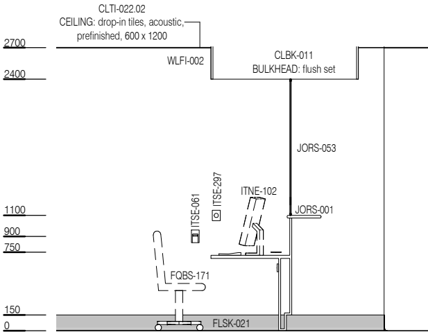
ELEVATION 1
