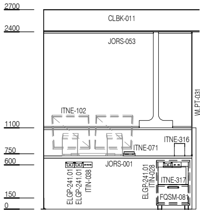
ELEVATION 2
