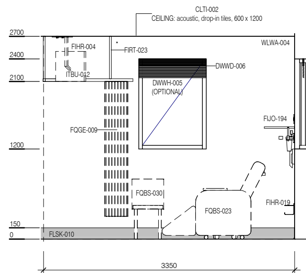
ELEVATION 2
