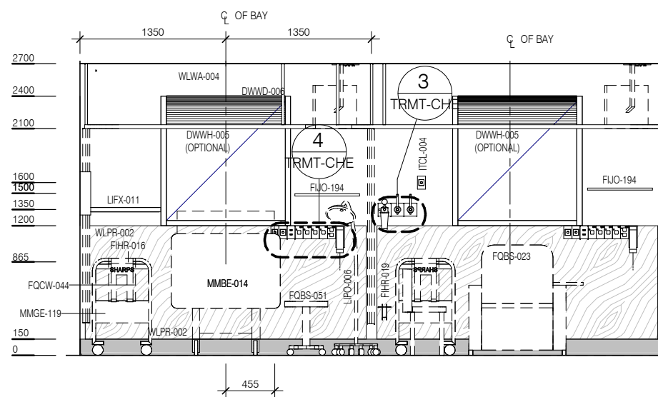
ELEVATION 1
