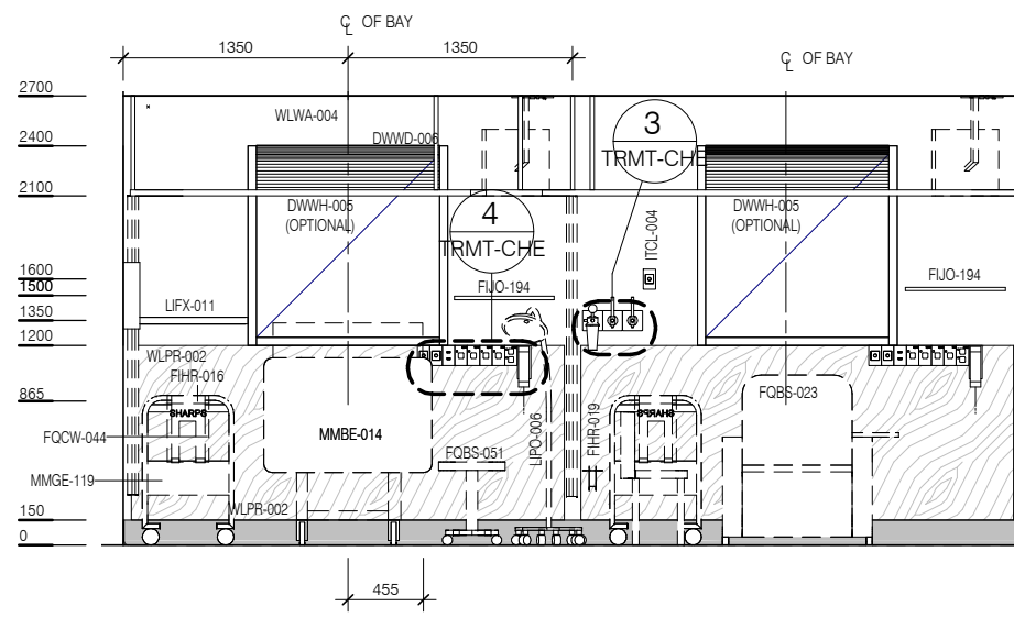
ELEVATION 1
