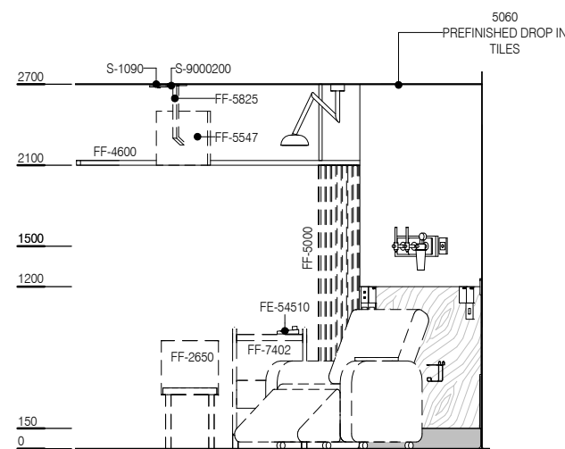
ELEVATION 2
