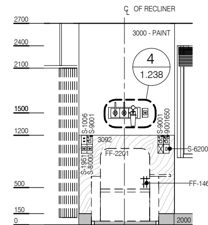
ELEVATION 3
