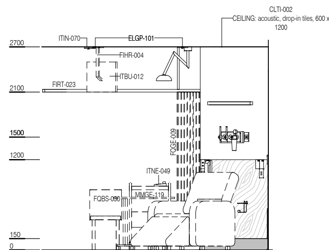
ELEVATION 2
