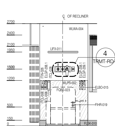
ELEVATION 3
