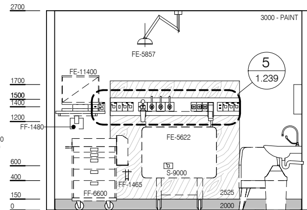
ELEVATION 2
