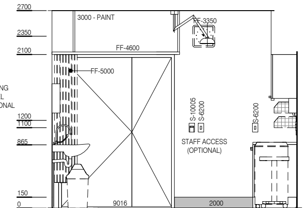
ELEVATION 4
