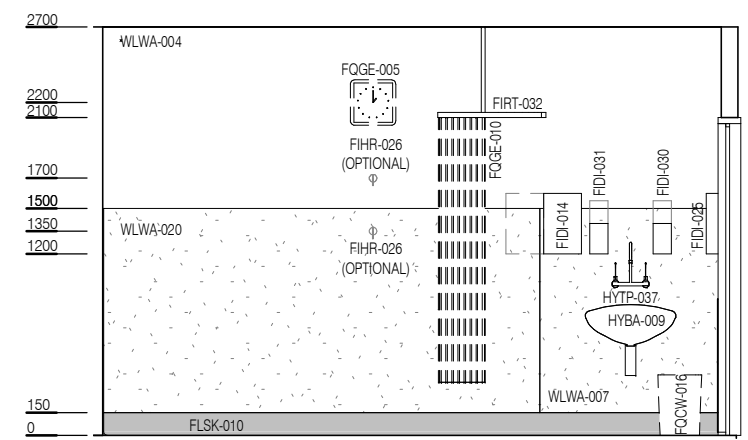
ELEVATION 2
