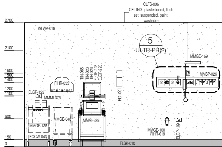
ELEVATION 1
