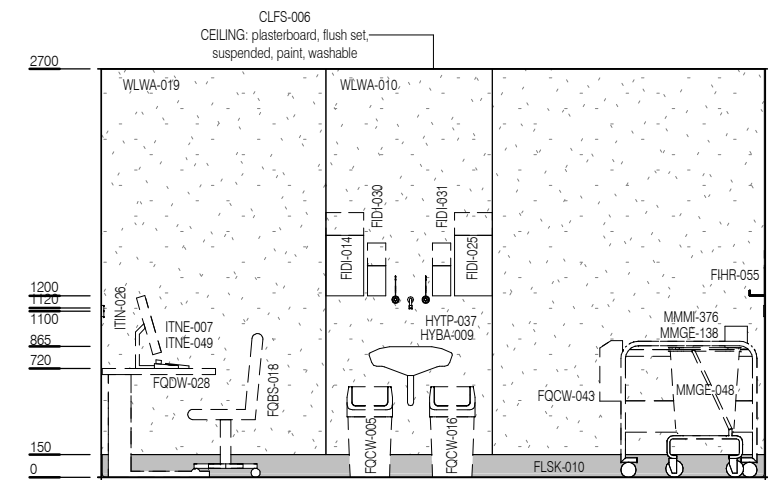
ELEVATION 4
