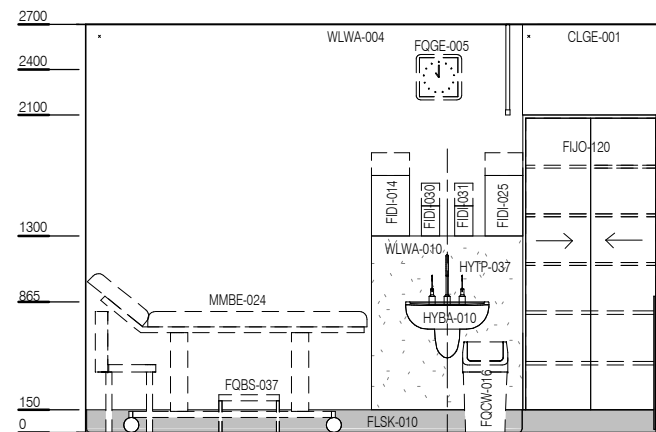
ELEVATION 2
