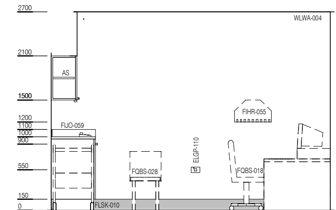
ELEVATION 4
