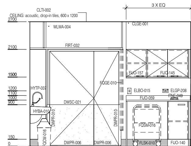
ELEVATION 3
