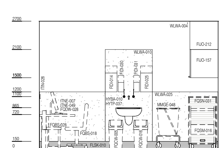
ELEVATION 4
