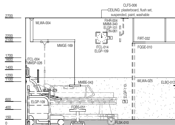
ELEVATION 2
