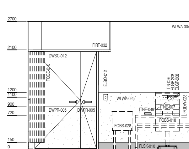
ELEVATION 3
