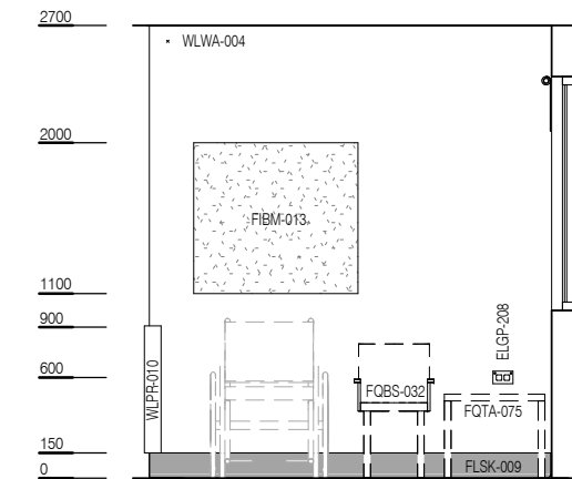
ELEVATION 3
