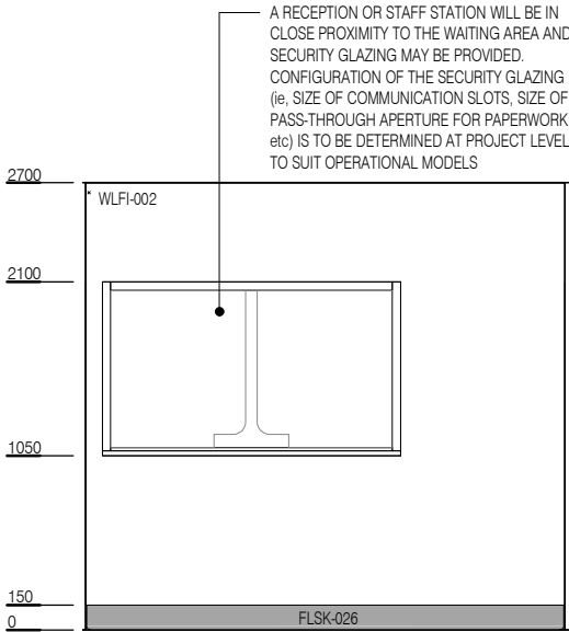
ELEVATION 2
