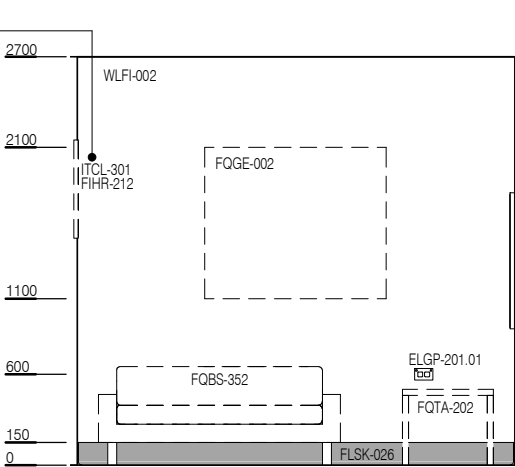
ELEVATION 4
