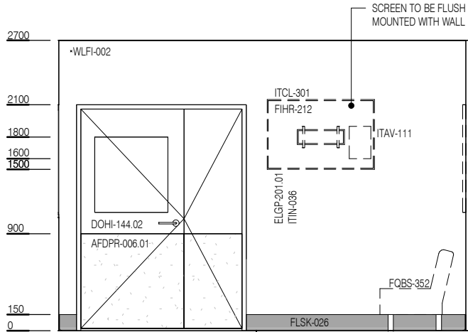
ELEVATION 3
