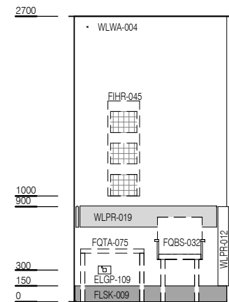
ELEVATION 2
