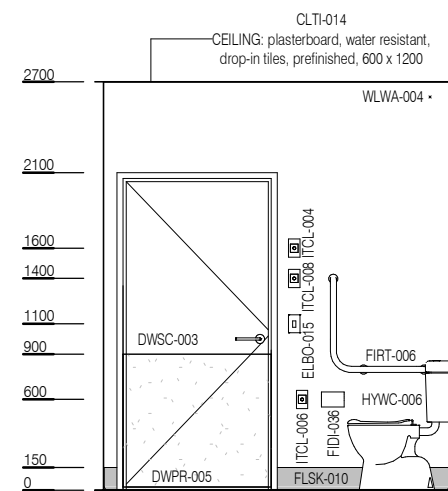
ELEVATION 2
