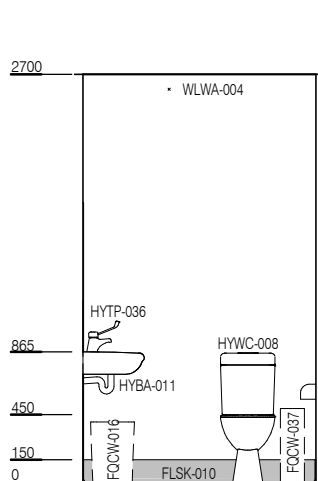
ELEVATION 1
